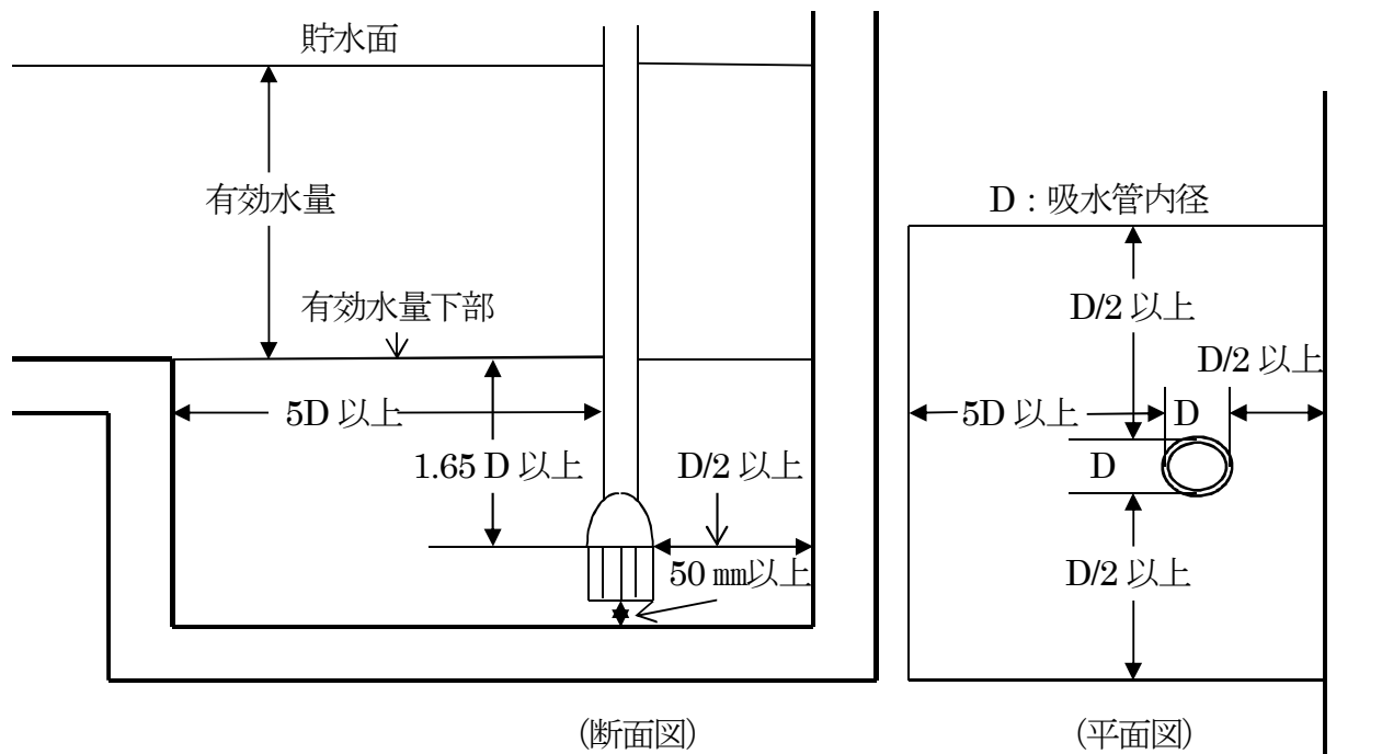
第2-7図 サクションピットを設ける場合の例
