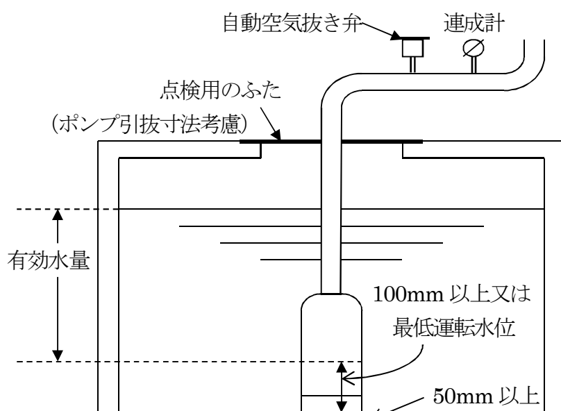
第2-10図 サクションピットを設けない場合
