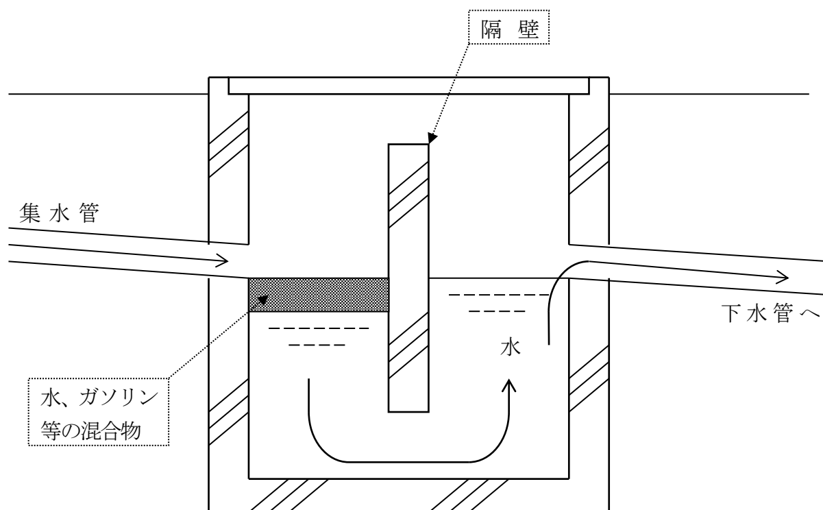
第5－3図 排水設備の構造例
