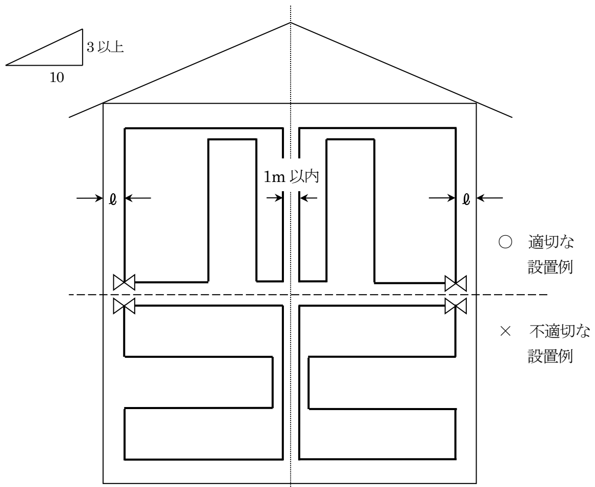
第 12-58 図 (断面図)
