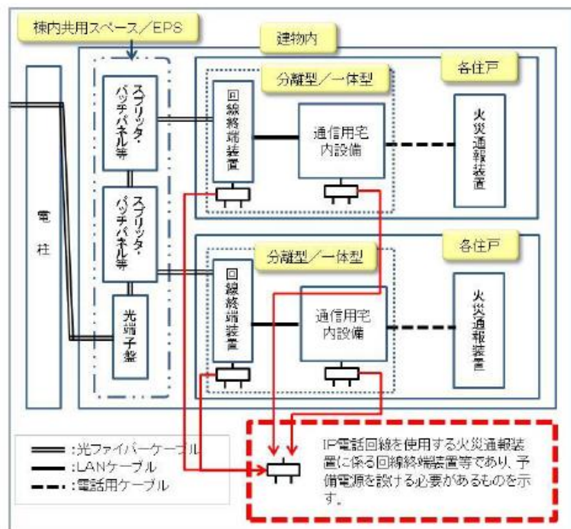
光配線方式
