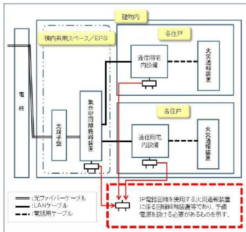
LAN 接続方式
