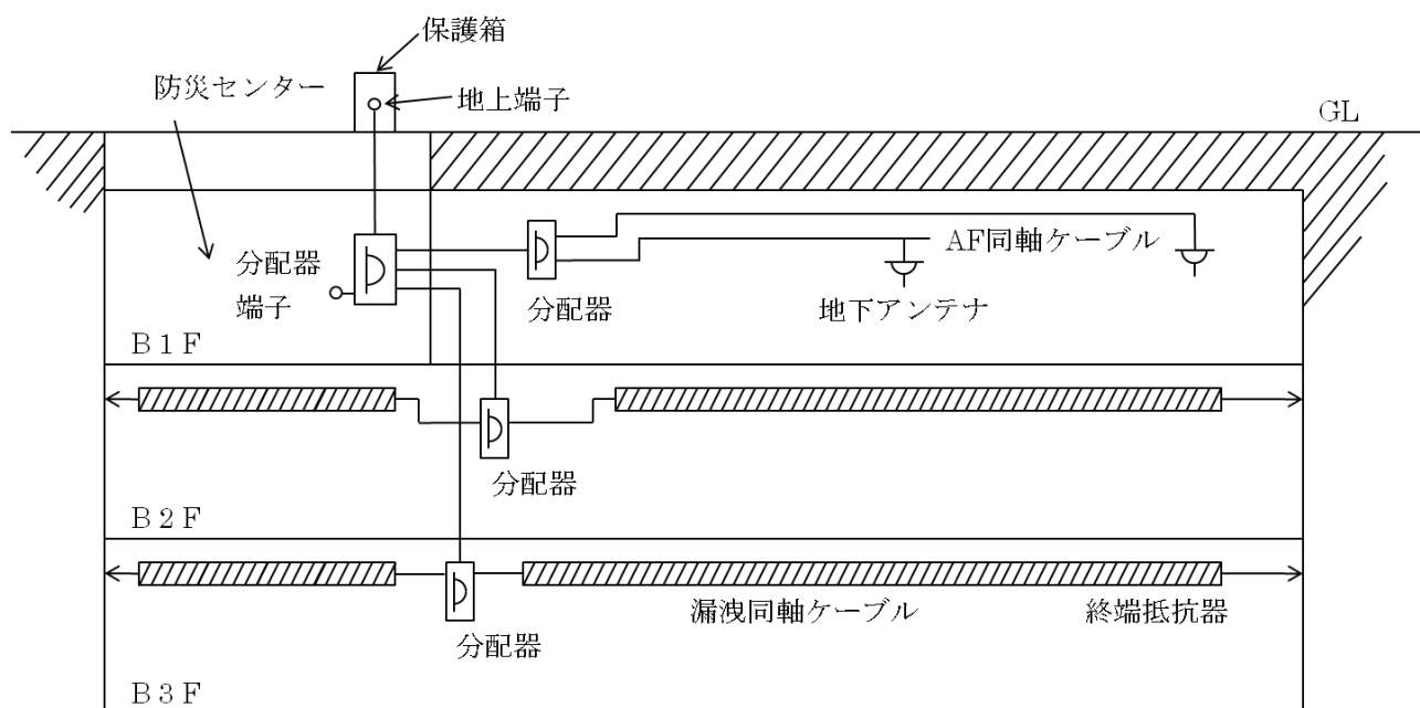
第 2 4－1 図 無線通信補助設備の構成例
