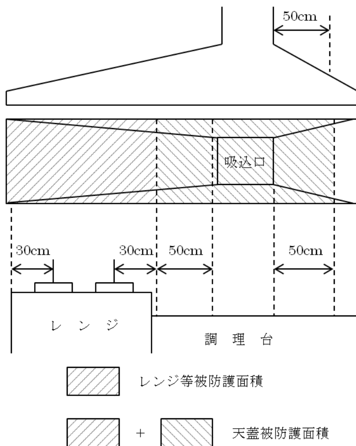
第 25-4 図 ダクト吸込口がレンジの直上部以外の位置にある場合の天蓋の被防護面積の例
