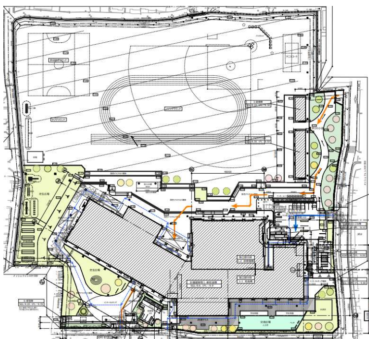
全体整備予定図
