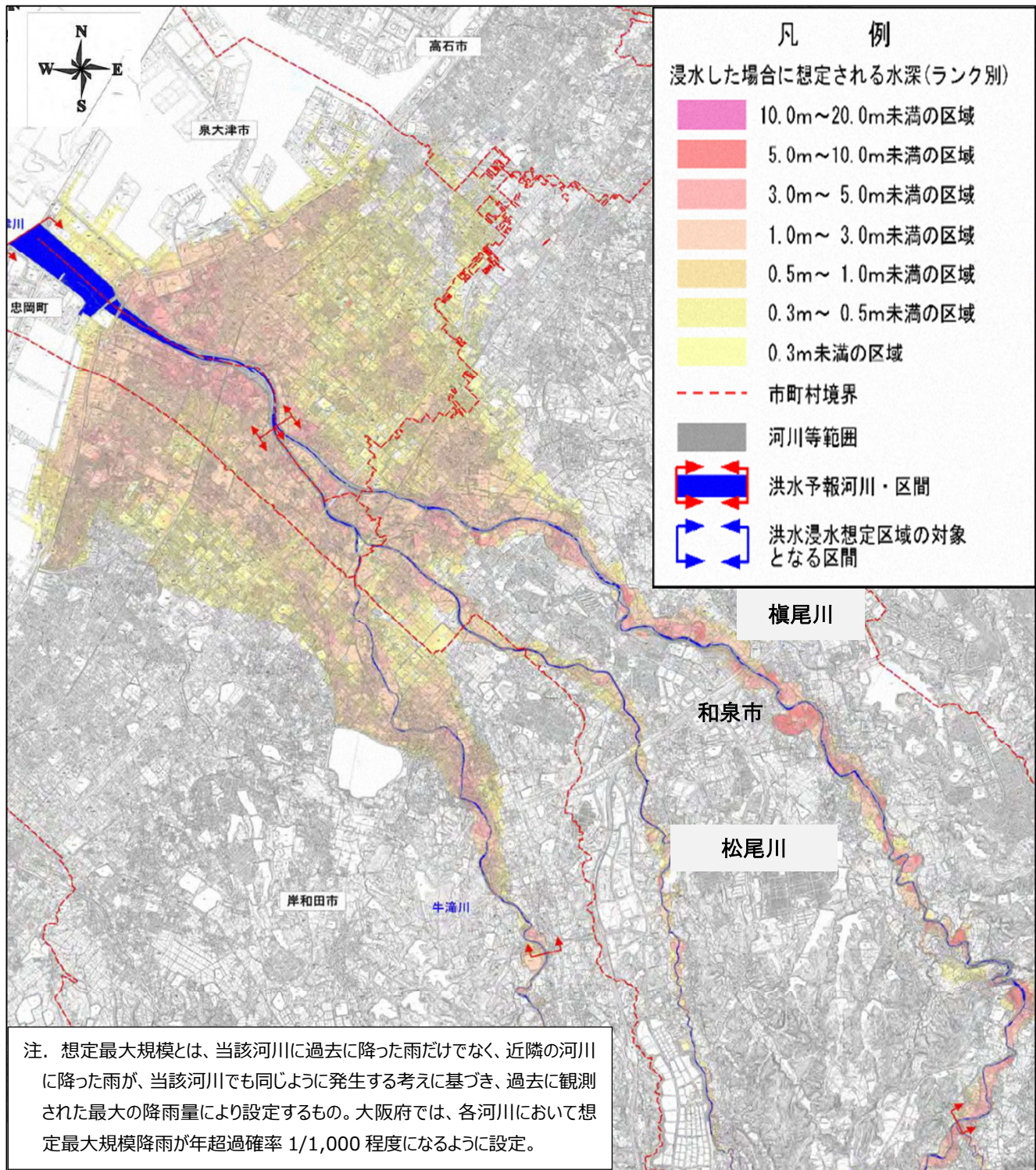
図 2.3.1 大津川水系大津川・榎尾川・東榎尾川・父鬼川・松尾川・牛滝川洪水浸水想定区域図
