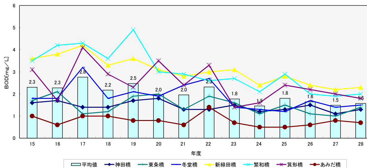
市内河川水質のBOD年平均値の推移
