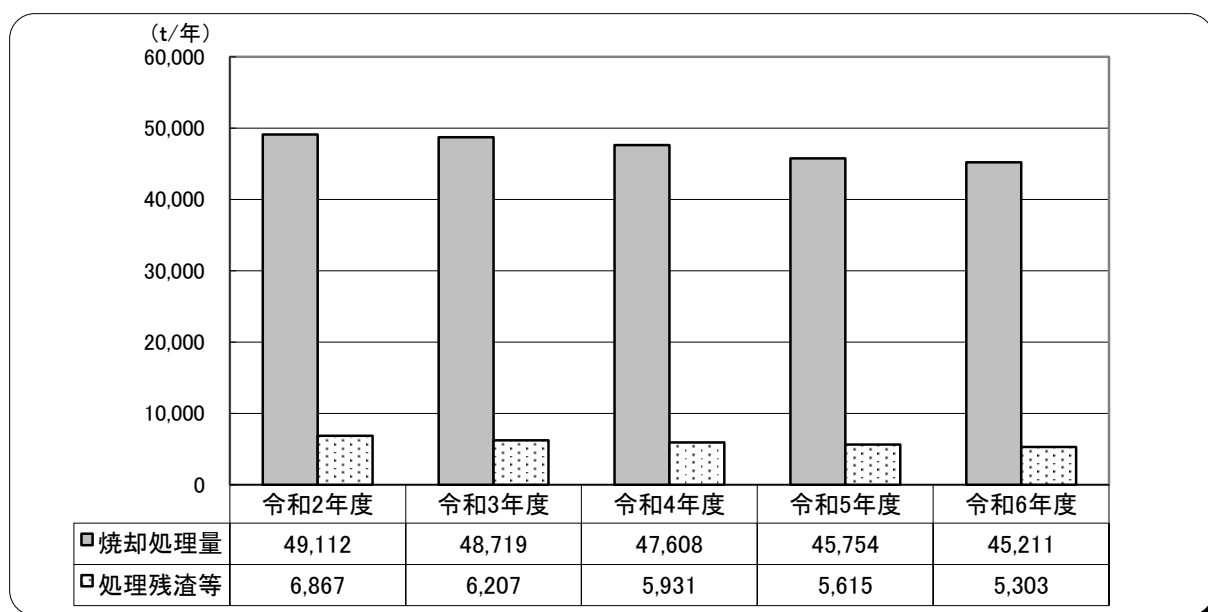
図 2-1-2 最終処分場施設の稼働実績の推移（組合）
