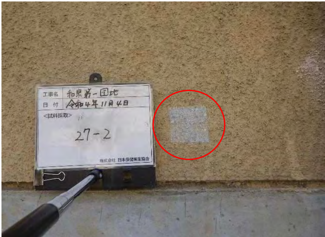
試料No.27 (採取後) 幸第二団地 49 棟 外壁 仕上塗材
