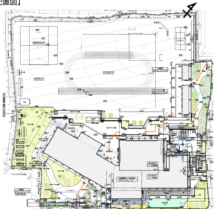
【配置図】
