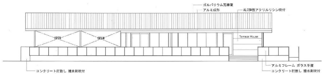
西立面図 1:100
