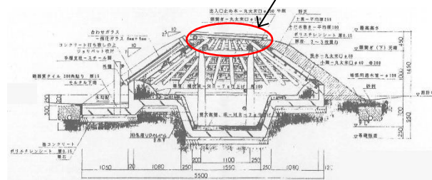
断面図
