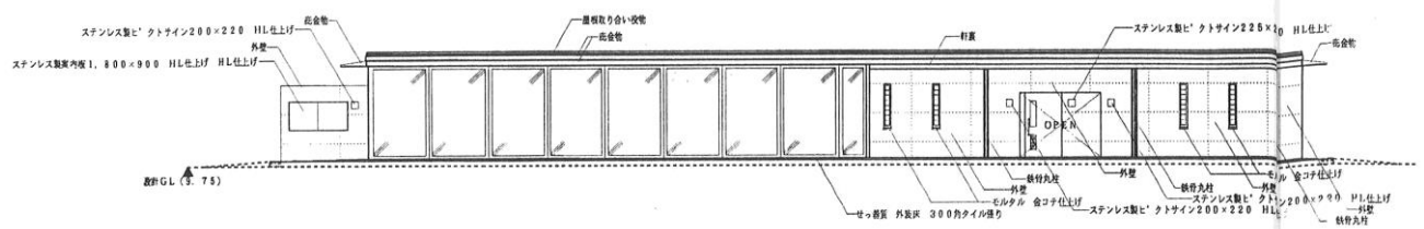
北立面図 S=1:100
