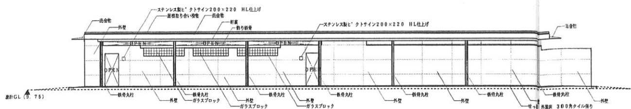
南立面図 S=1:100
